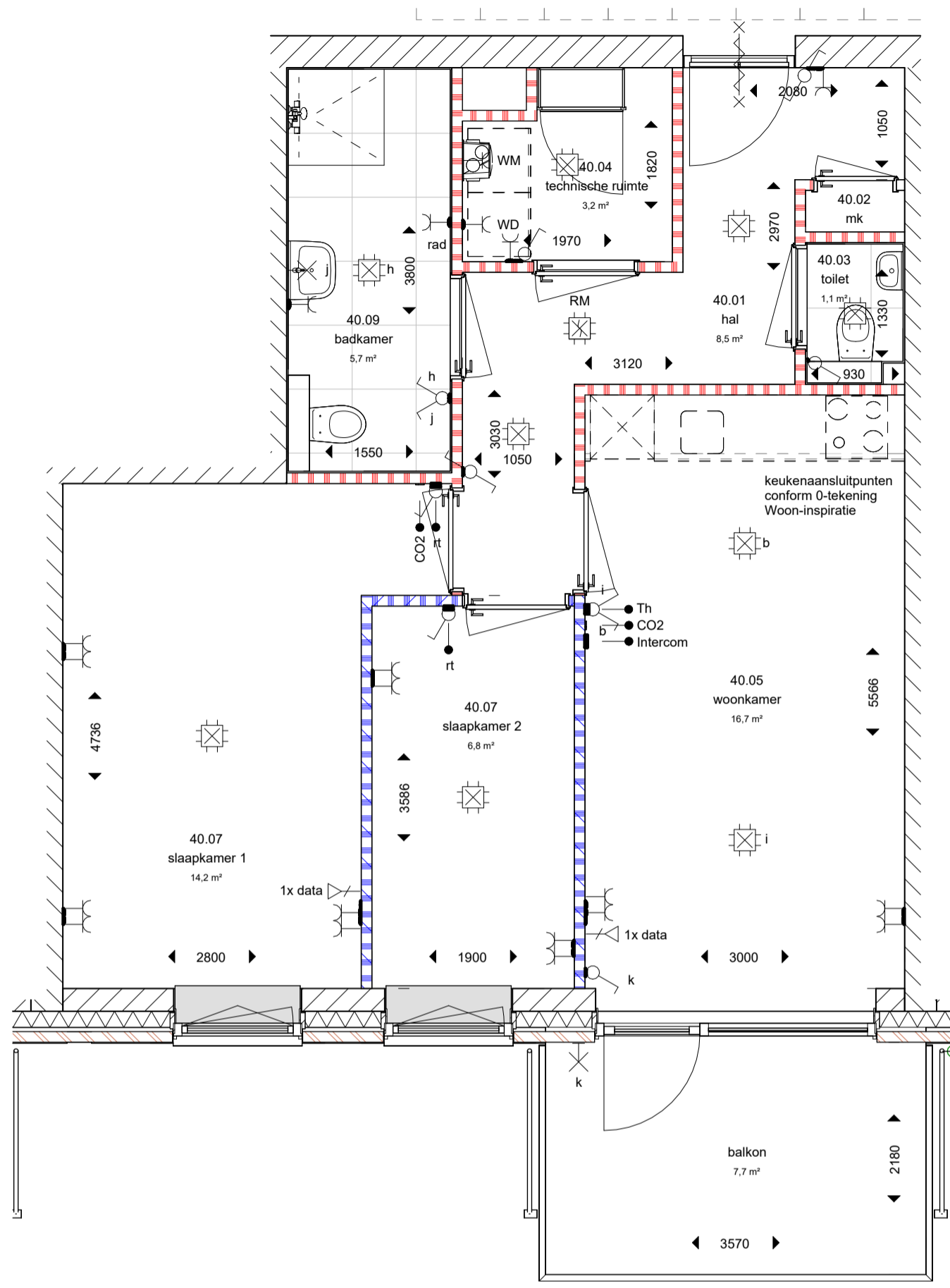
bnr 40 - type (B) 1 : 50
