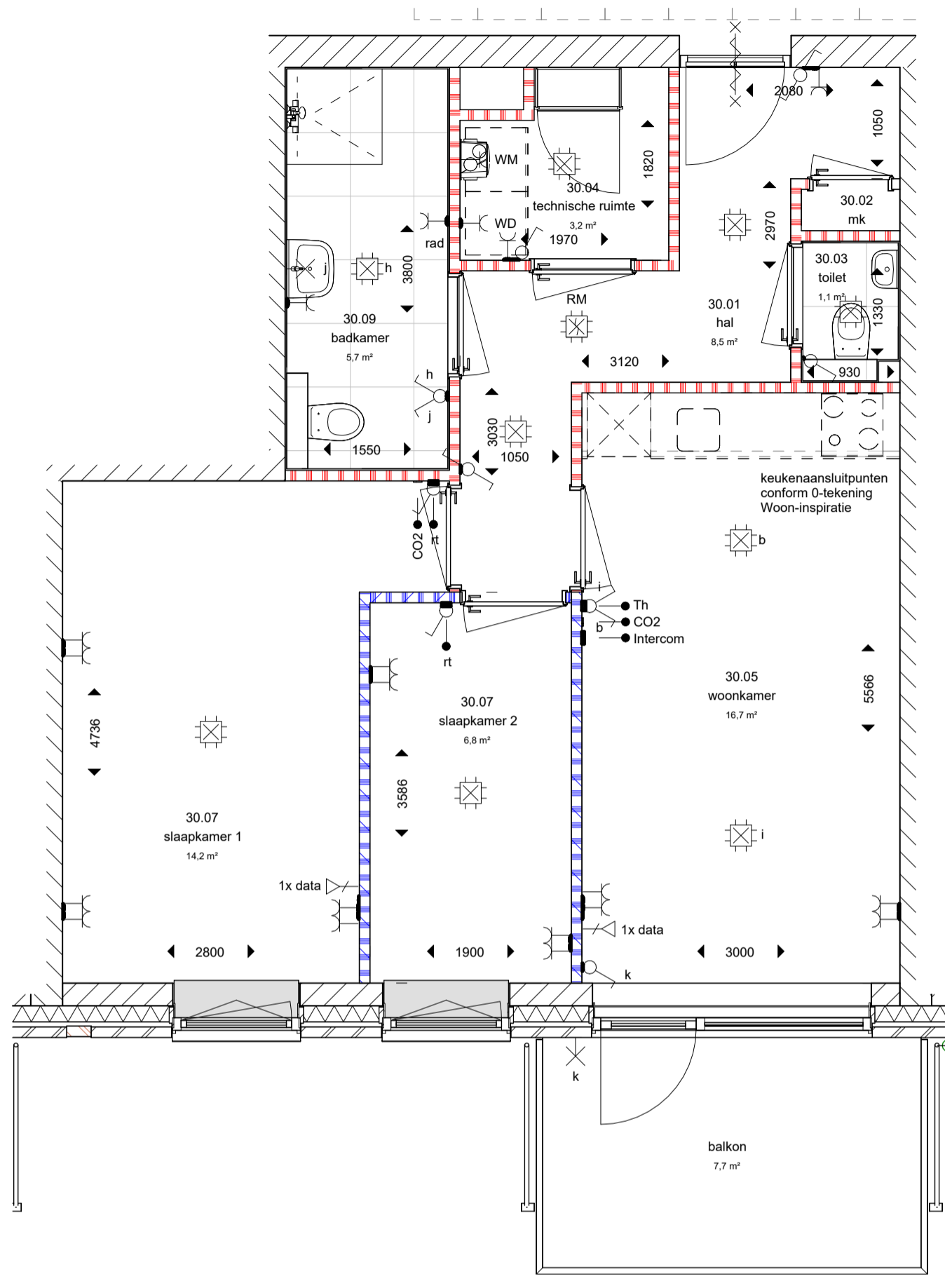
bnr 30 - type (B) 1 : 50
