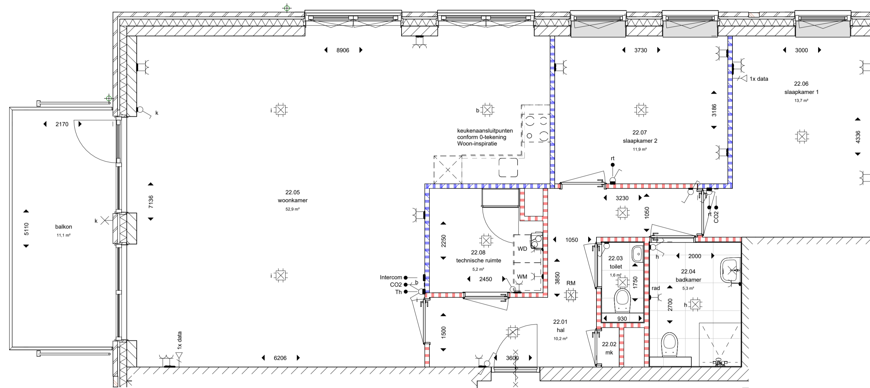
bnr 22 - type (D) 1 : 50
