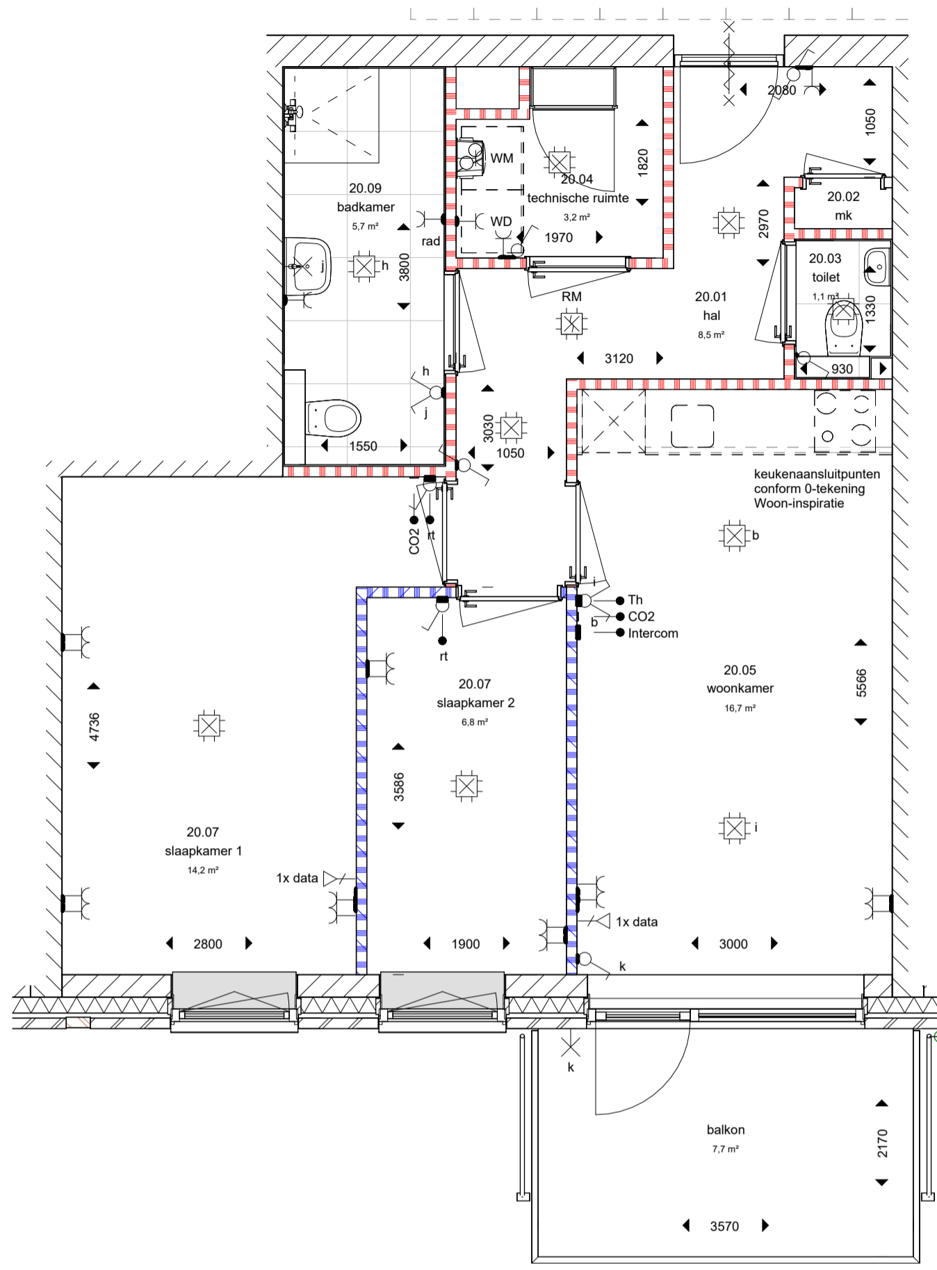
bnr 20 - type (B) 1 : 50
