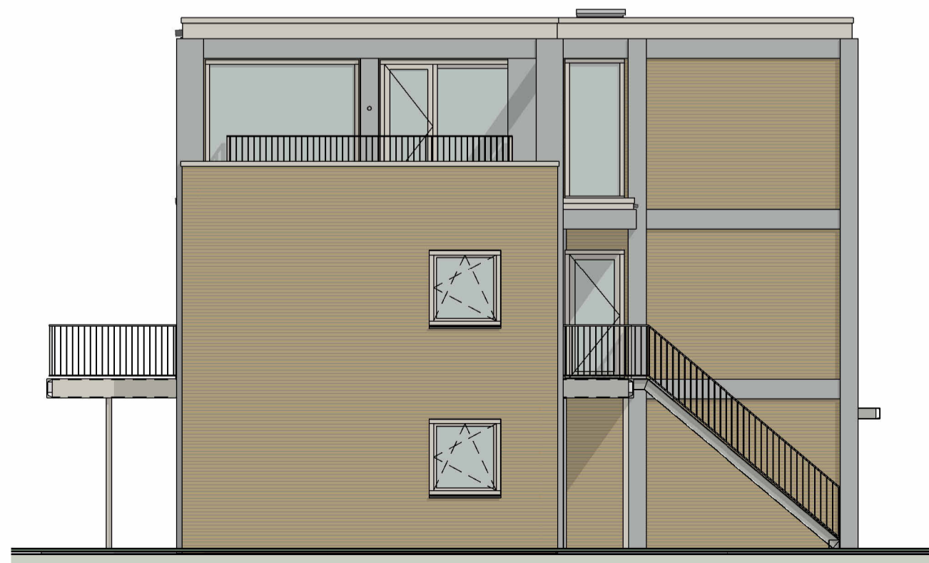
linkergevel (gebouw C)
