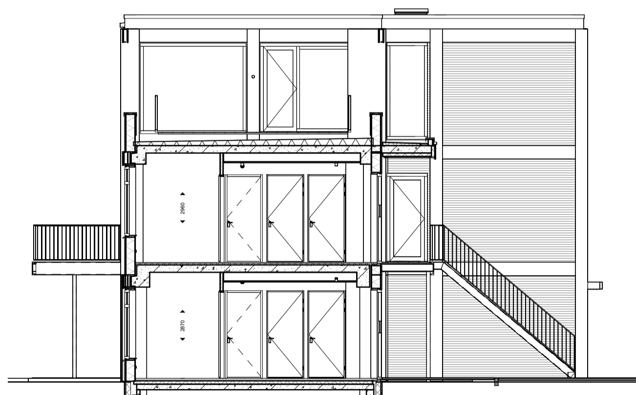
doorsnede 2-2
