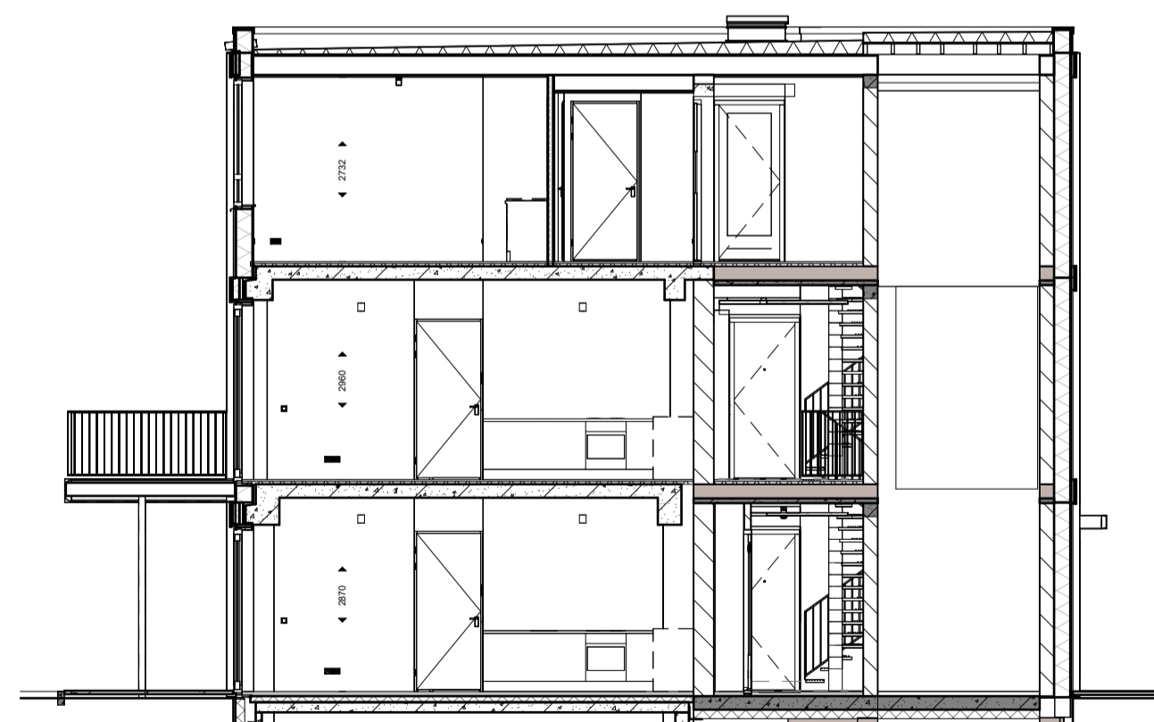
doorsnede 3-3
