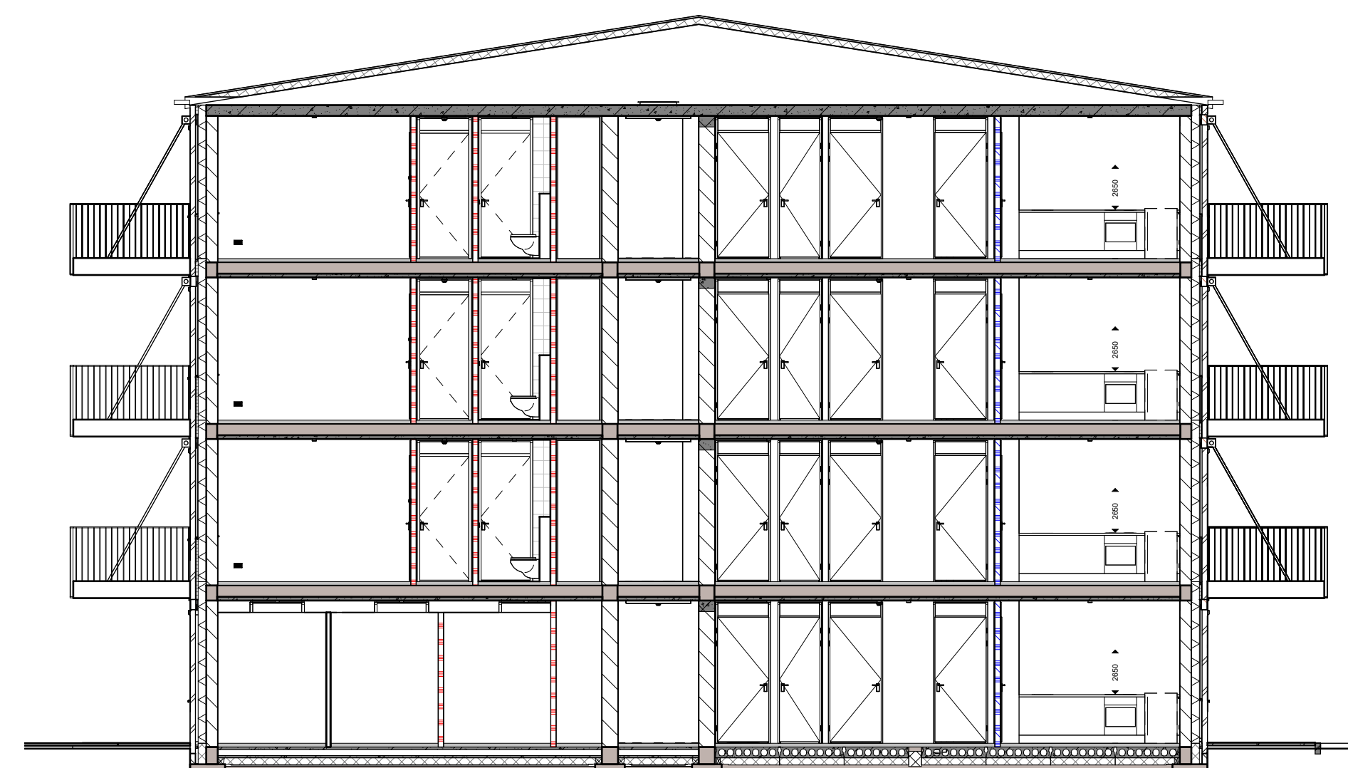
doorsnede B-B
